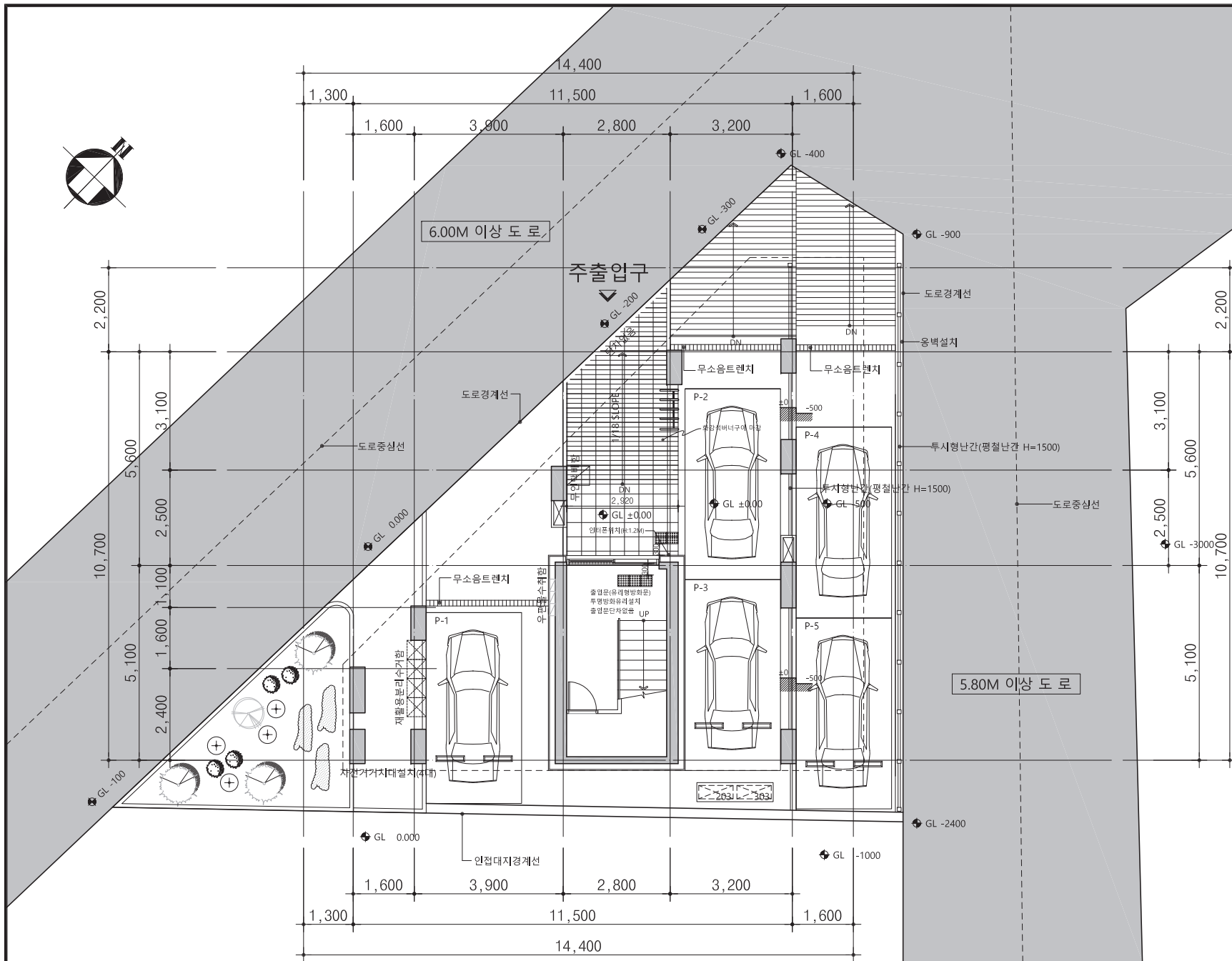
1 층 평 면 도 축척: 1/ 100
